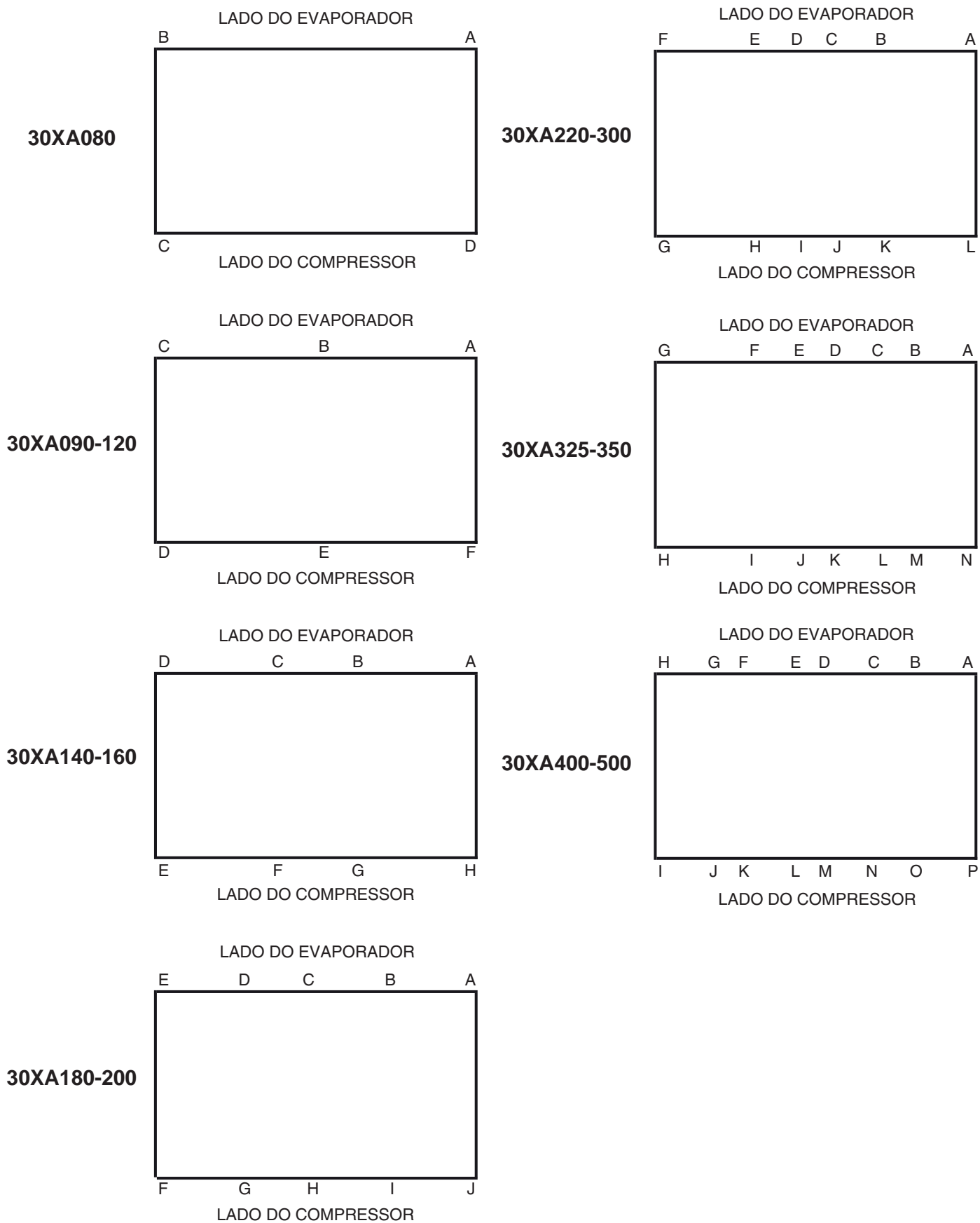
Fig. 1b - Pesos de montagem da unidade (unidades com serpentina condensadora Al/Cu)
