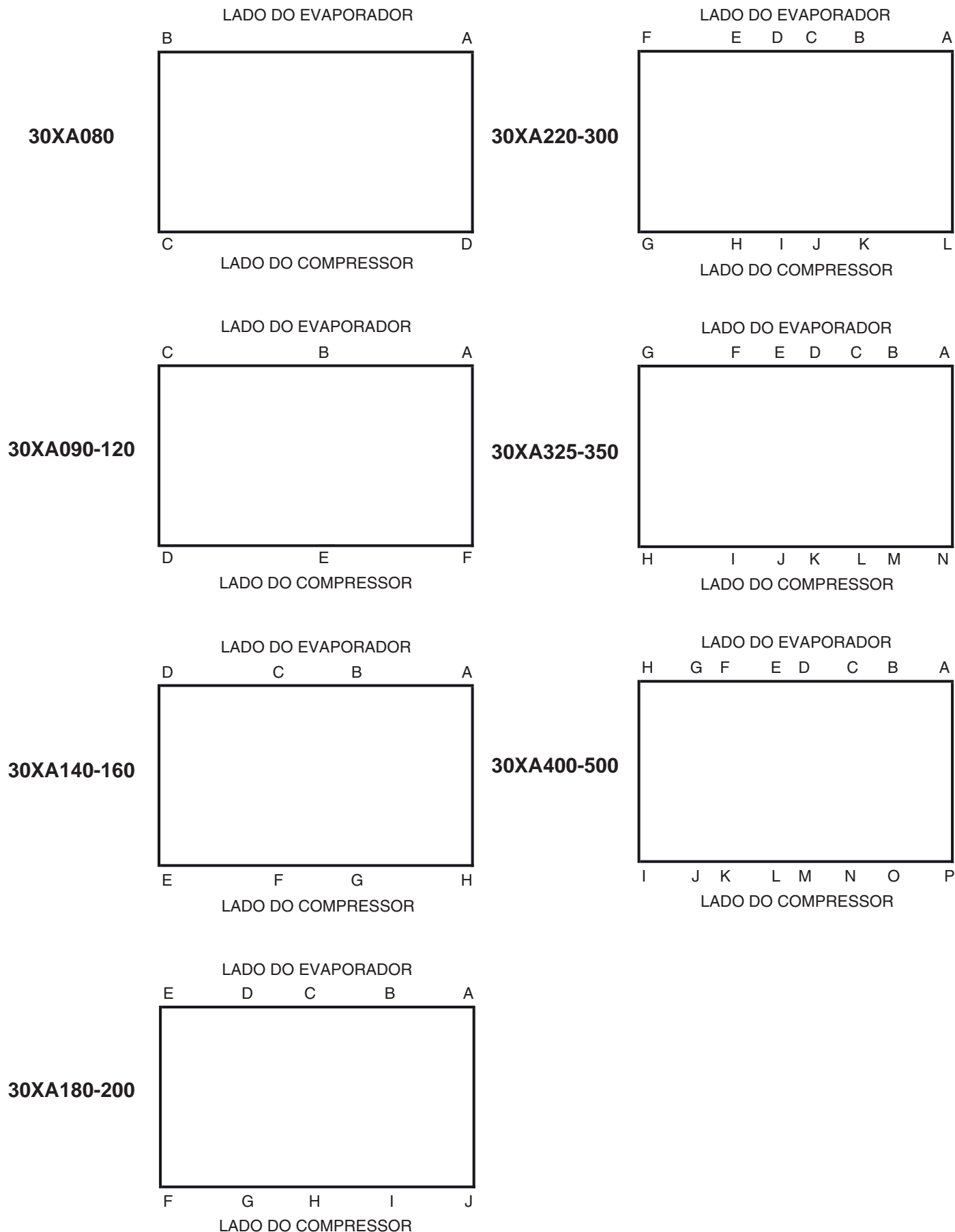
Fig. 1d - Pesos de montagem da unidade (unidades com serpentina condensadora MCHX)
