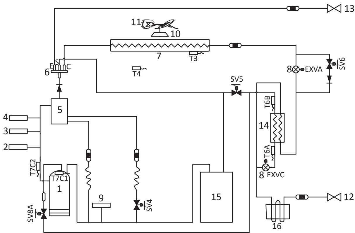
Figura 2-4.1: Diagramas de tubulação 8/10/12HP
