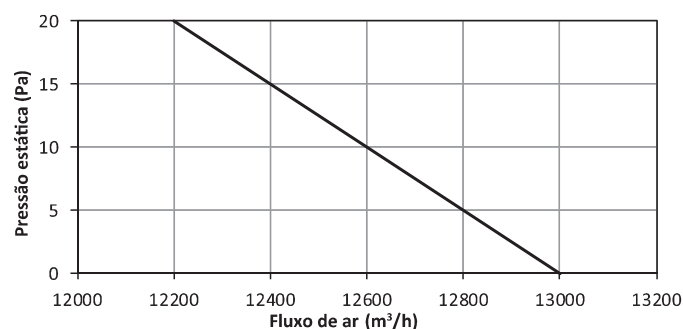
Figura 3-3.10: Desempenho de ventilador das unidades de 14-18HP
