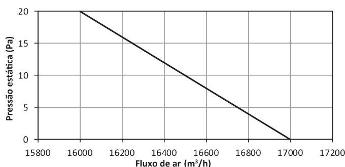
Figura 3-3.11: Desempenho de ventilador das unidades de 20-22HP
