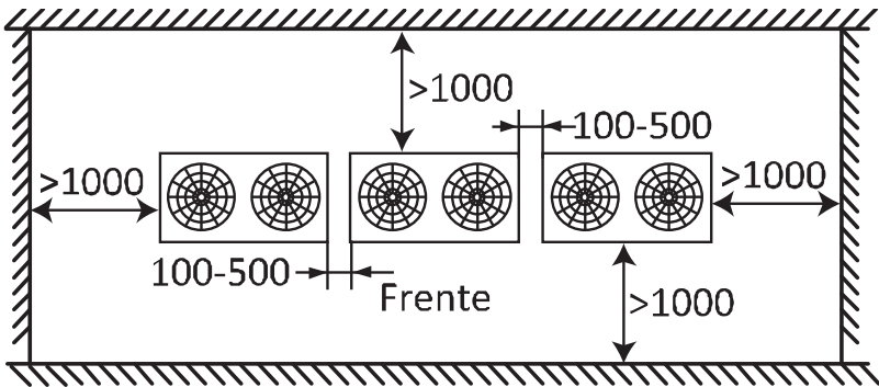
Figura 2-3.2: Instalação de unidades em filas (unidade: mm)
