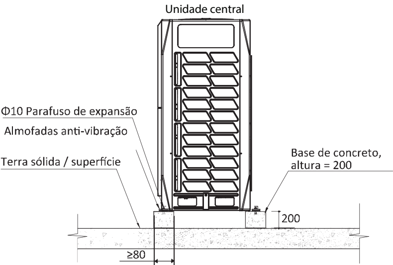
Figura 3-2.4: Projeto da estrutura de base de concreto típico da unidade central (unidade: mm)
