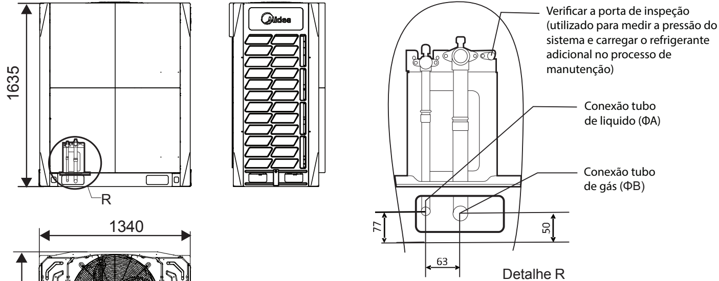
Figura 2-2.2: Dimensões 14/16/18HP (dimensões em mm)
