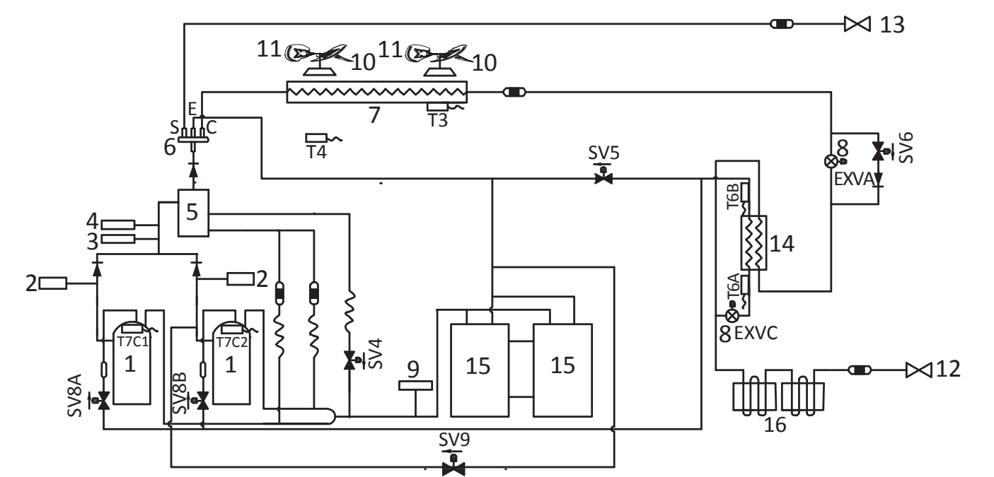
Figura 2-4.4: Diagramas de tubulação 26/28HP
