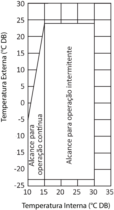
Figura 2-9.2: Limites de operação de aquecimento
