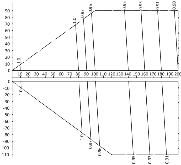
Figura 2-8.2: Taxa de mudança na capacidade de aquecimento
