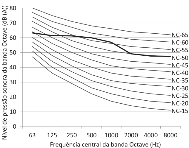
Figura 2-10.5 Nível da banda de oitava de 18HP
