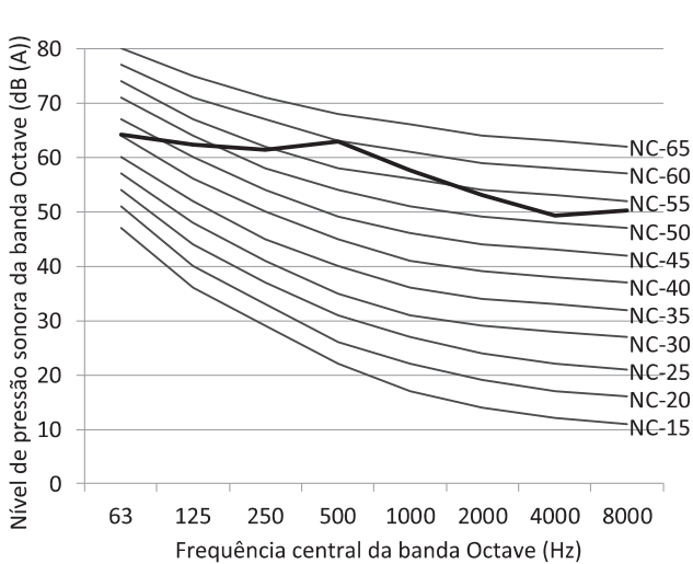
Figura 2-10.6 Nível da banda de oitava de 20/22HP
