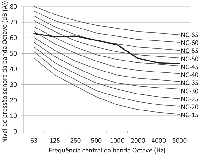
Figura 2-10.3 Nível da banda de oitava de 12/14HP
