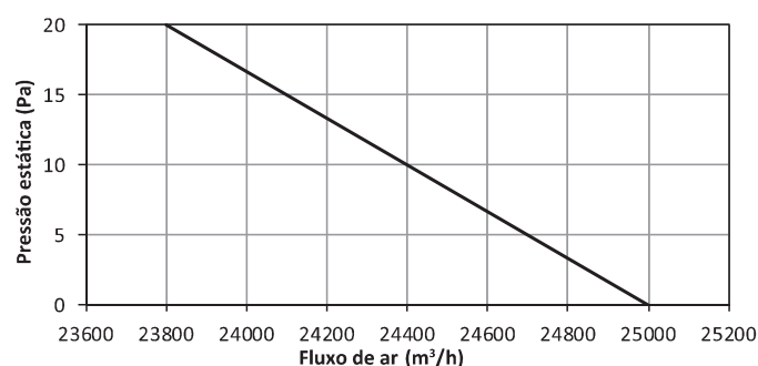
Figura 3-3.12: Desempenho de ventilador das unidades de 24-28HP
