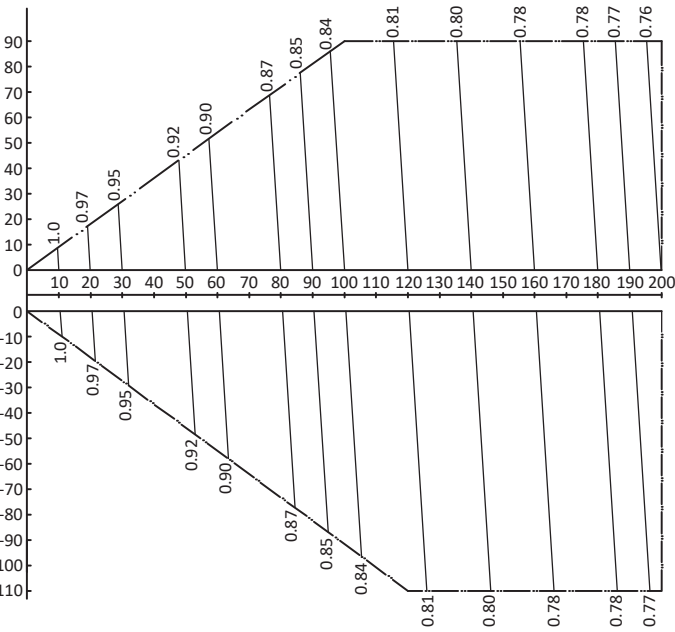
Figura 2-8.1: Taxa de mudança na capacidade de refrigeração
